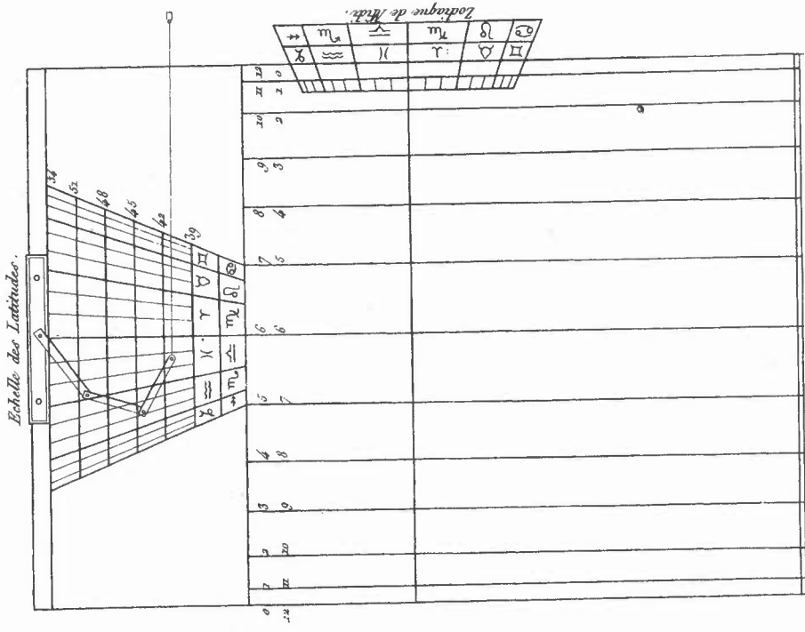
Fig. 74. Analemme Rectiligne universel.
